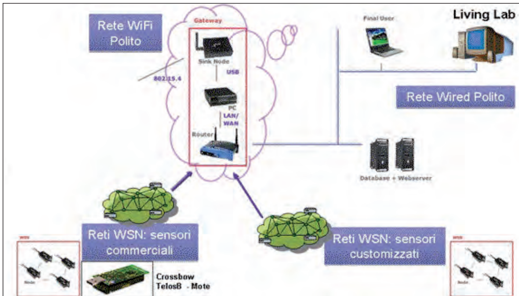
Figura 2. Sistema Integrato di Monitoraggio (SIM): schema logico e componenti.
