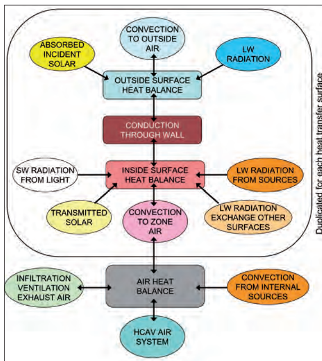
Figura 4. Schema concettuale del modello termoeconomico di un edificio.
