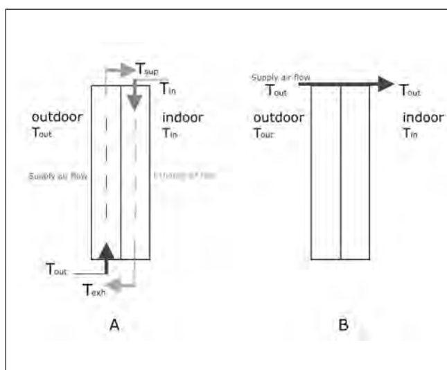
Figura 8. A: schema di funzionamento di una finestra "dual air flow"; B: finestra tradizionale.
