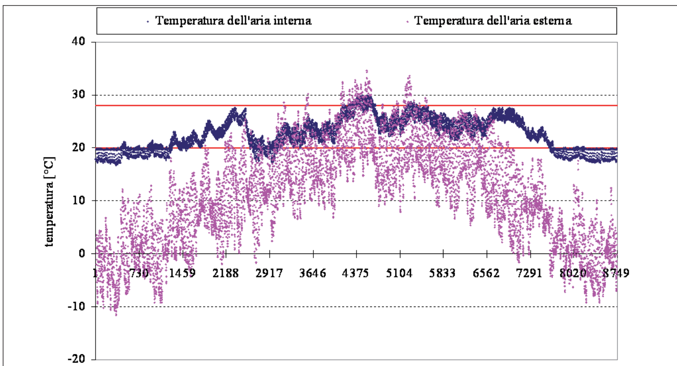
Figura 1. Valutazione lungo un intero anno (8760 ore) della temperatura dell'aria interna in un edificio passivo montano con indicazione delle temperature dell'aria esterna e della banda di accettabilità della temperatura interna (in rosso)(da E. Fabrizio, M. Filippi, Sistema multienergia per un edificio a energia netta zero in clima alpino , 64° Congresso ATI, L'Aquila - Montesilvano (PE), 8-11 settembre 2009, paper 4.15).
