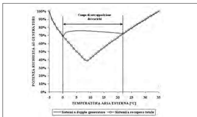
Figura 17. Potenza richiesta ai generatori. I sistemi a recupero totale richiedono minor potenza rispetto ai sistemi a doppio generatore nel campo della sovrapposizione dei carichi.
