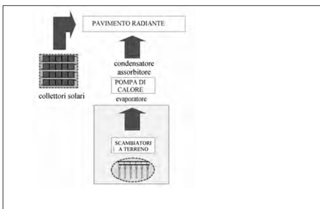
Figura 19. Pompa di calore ad assorbimento di un sistema Total Energy che utilizza l'aria espulsa come sorgente termica nel funzionamento invernale.
