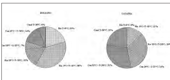
Figura 24. Richiesta di energia per fasce di temperatura (edificio ad uso alberghiero).
