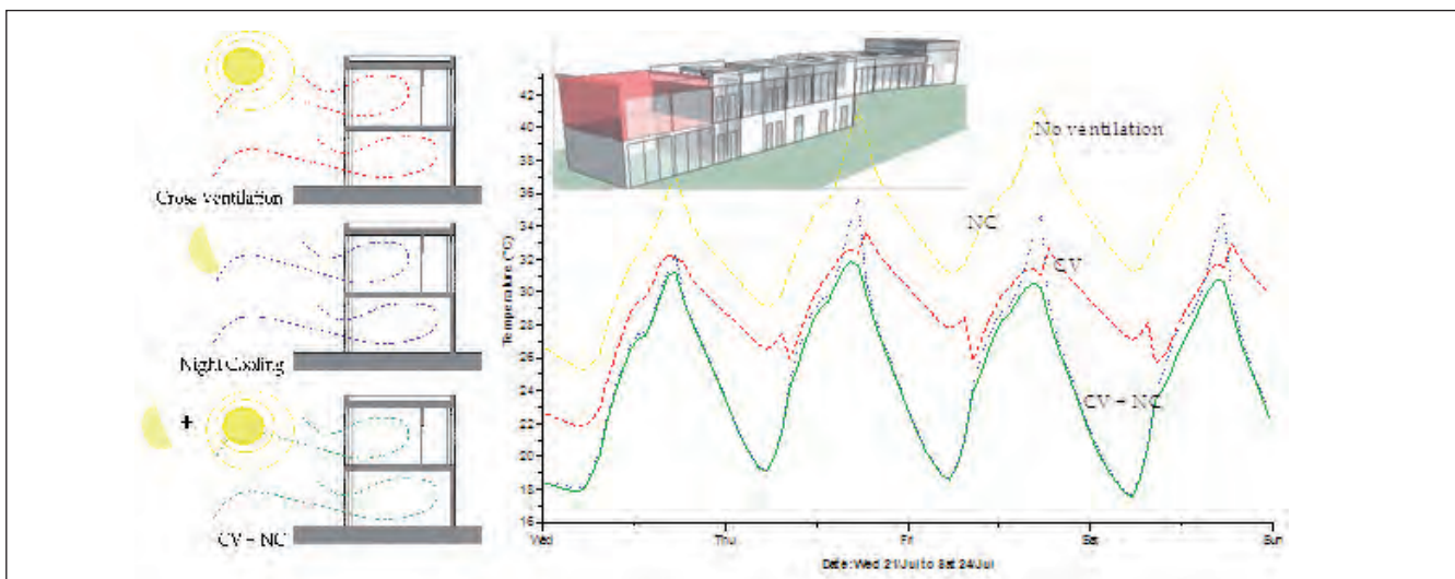
Figura 9. Valutazione del comfort termico ambientale estivo per le diverse strategie di ventilazione.
