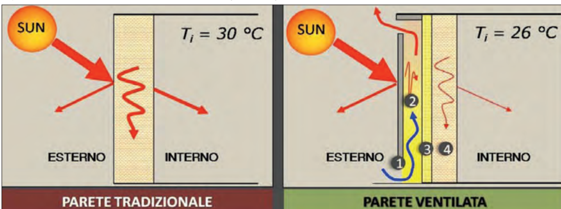
Figura 4. Trasmissione del calore attraverso componenti opachi di involucro.
