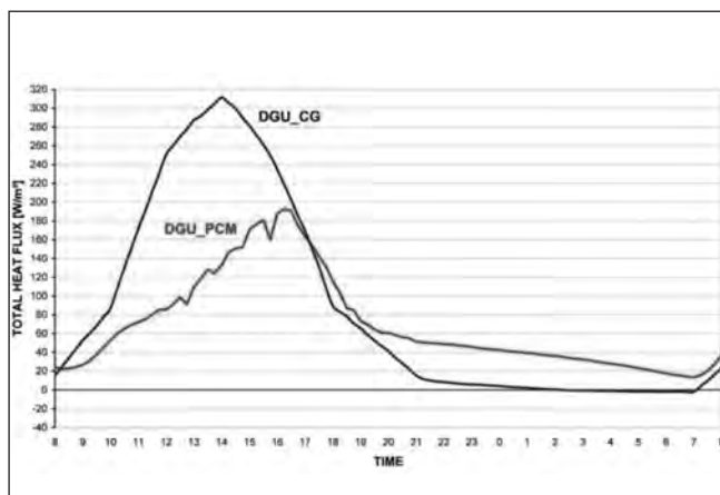
Figura 10. Flussi termici totali attraverso un vetro camera tradizionale ed una vetratura con PCM.
