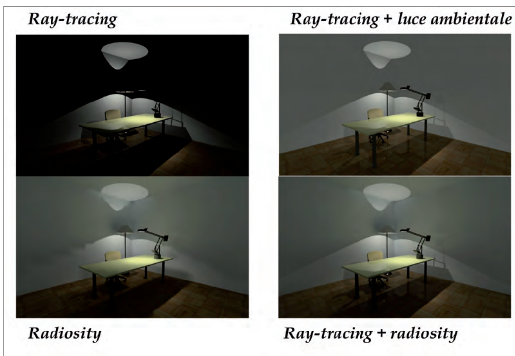
Figura 5. Esempi di applicazione degli algoritmi di radiosity e raytracing o di combinazione di diversi algoritmi.
