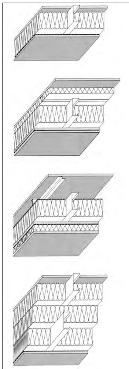
Figura 1. Solaio in legno: assonometria di un tipico sistema costruttivo assemblato a secco in legno (fonte: Lignatur).
