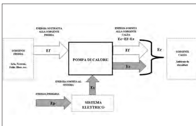
Figura 8. Bilancio energetico di un sistema a pompa di calore in termini di energia primaria.
