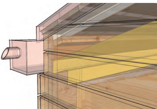
Figura 8. Dettaglio della gronda.
