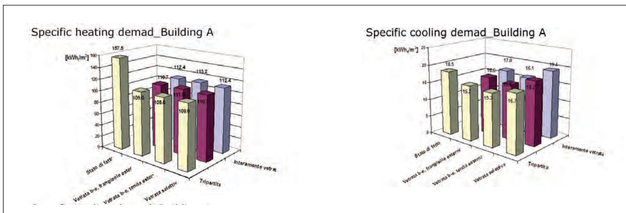
Figura 3. Risultati dei calcoli, differenze tra l'energia sensibile per il riscaldamento e il raffrescamento. Figura 4. Risultati dei calcoli, fabbisogno specifico di energia per il riscaldamento e il raffrescamento, edificio A.
