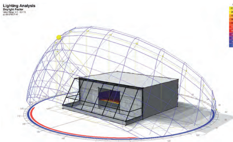
Figura 8. Studio dell'illuminazione naturale con Ecotect. Dinamica delle ombre prodotte dalla radiazione solare diretta e distribuzione del fattore di luce diurna.
