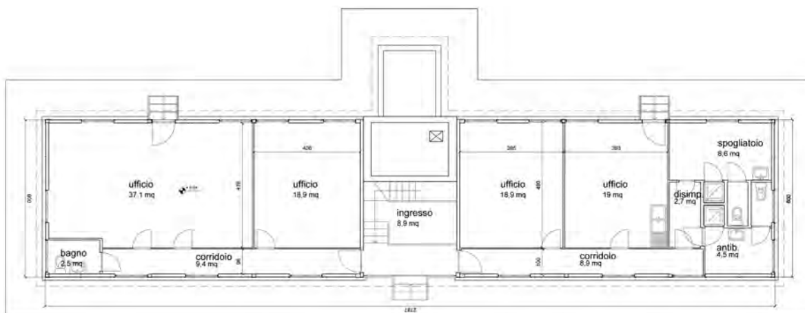
Figura 4. Pianta dello stato di fatto.
