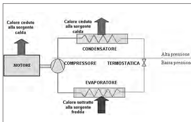
Figura 3. Sistema Total Energy nella configurazione più semplice.
