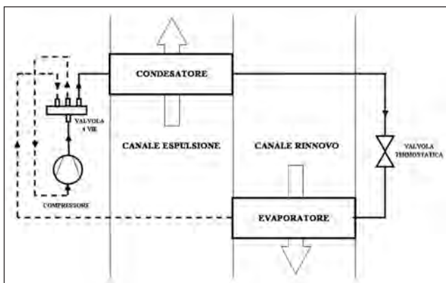
Figura 18a. Recupero tramite pompa di calore a compressione (funzionamento estivo).
