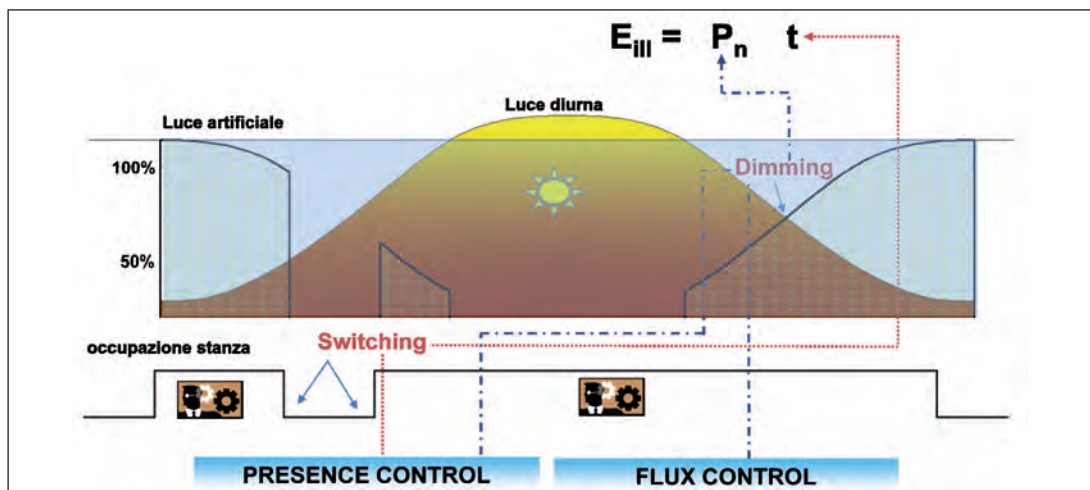
Figura 5. Esempio di controllo dei livelli di illuminazione naturale e artificiale in un ambiente.
