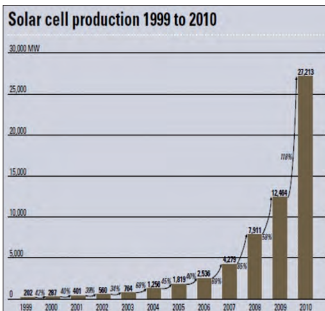
Figura 2. Andamento della produzione di celle solari dal 1999 al 2010.
