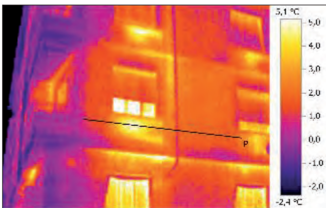
Figura 5. Termografia all'esterno del fabbricato.
