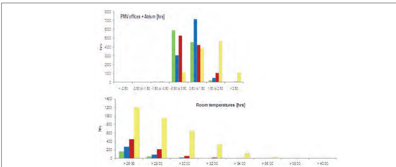
Figura 9. Valutazione del comfort termico ambientale estivo per le diverse strategie di ventilazione.
