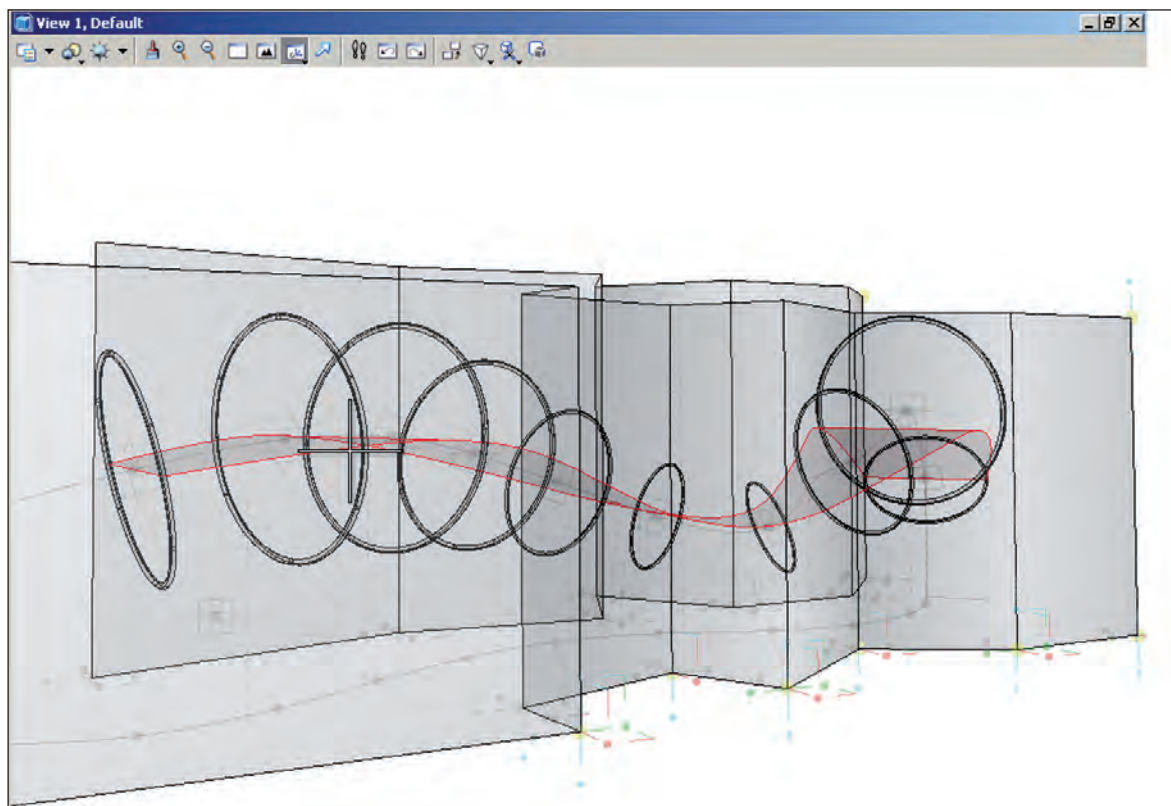
Figure 8a, 8b. Progetto di passerella parametrica in contesto urbano con Generative Components.
