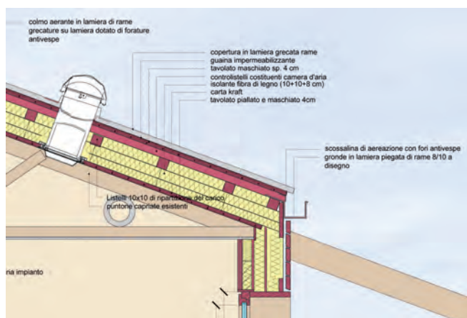
Figura 15. Sezione del raccordo tra tetto e parete.
