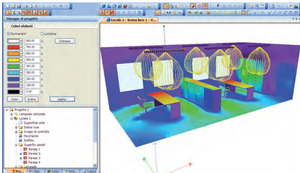
Figura 7. Interfaccia DIALux nella fase di visualizzazione in false color dei risultati di illuminamento sulle superfici.
