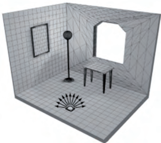
Figura 3. Schema concettuale dell'algoritmo di radiosity.
