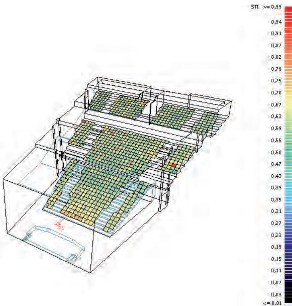
Figura 3. Esempio di mappa colorimetrica per la valutazione della distribuzione dei parametri di qualità acustica (ie: indice di intelligibilità STI) all'interno della sala, ottenibile dalla simulazione al calcolatore attraverso l'impiego del software Odeon.
