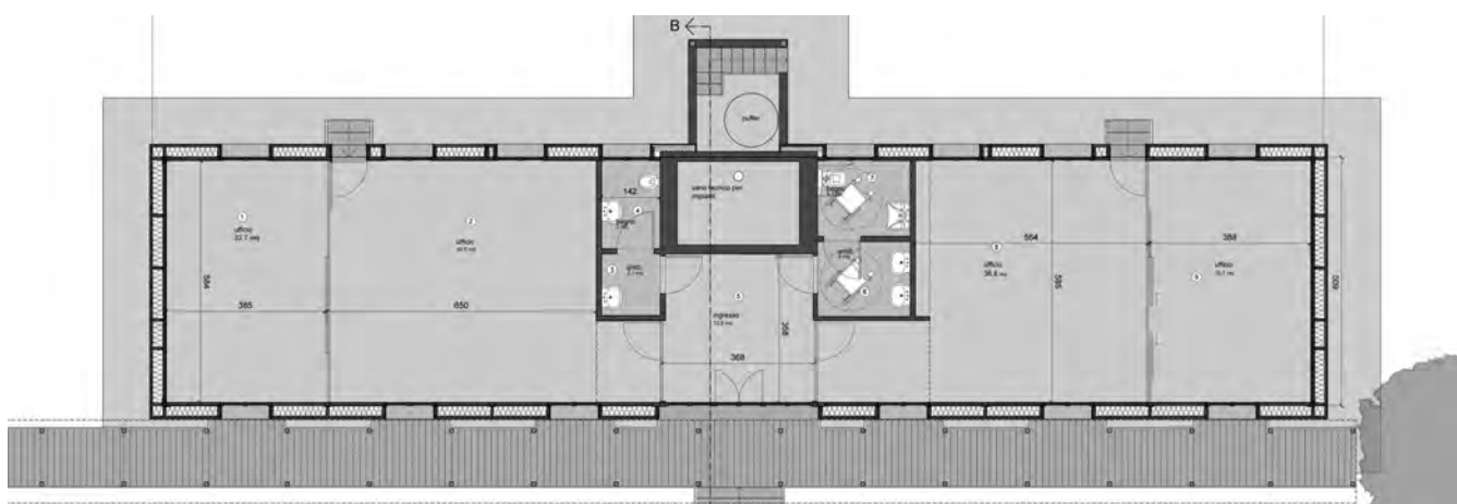
Figura 5. Pianta di progetto.
