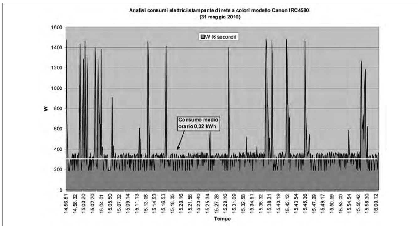
Figura 13. Acquisto di macchine da ufficio con criteri di sostenibilità. Rilievi delle prestazioni energetiche.
