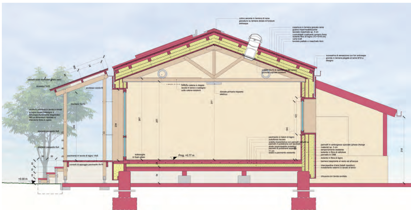
Figura 6. Sezione di progetto.
