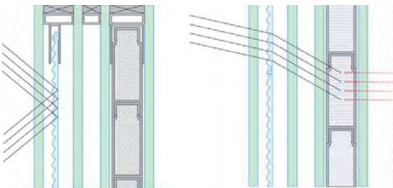
Figura 7. Facciata con pannelli prismatici e PCM (fonte: GlassX, CH).
