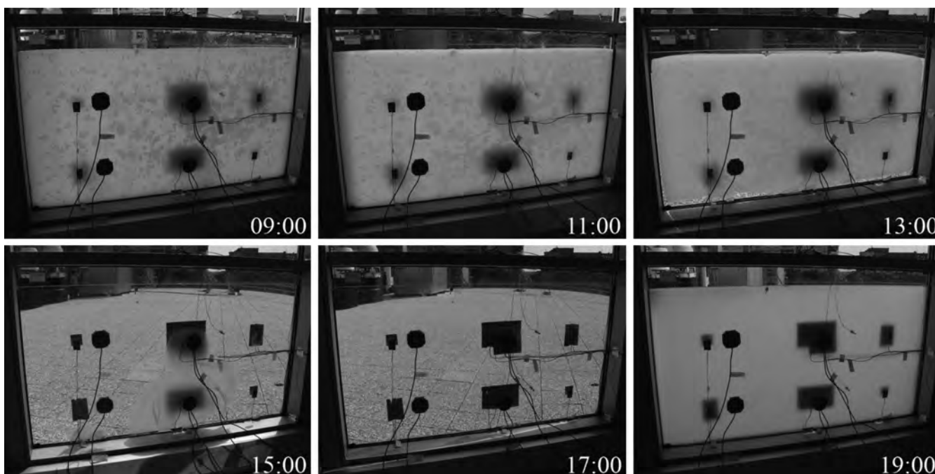
Figura 11. Comportamento di un prototipo sperimentale di vetrocamera con PCM durante una giornata estiva con elevato irraggiamento solare.
