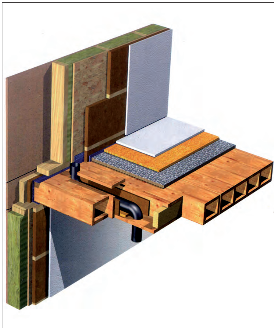
Figura 2. Stratigrafie SR: assonometrie di alcune soluzioni di involucro in struttura metallica leggera e lastre di completamento (fonte: Stahl-Information-Zentrum).
