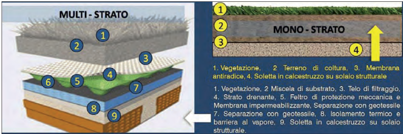
Figura 2. Verde pensile estensivo ed intensivo.
