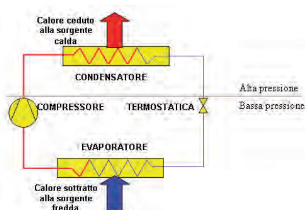
Figura 2. Circuito frigorifero a compressione.
