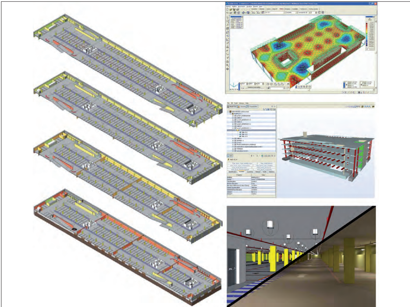
Figura 3. Esploso assometrico, verifiche strutturali e illuminotecniche del modello parametrico realizzato per il progetto preliminare del parcheggio interrato pluripiano presso la Cittadella Politecnica. Autori: G. Cangialosi e M. Lo Turco (2008).
