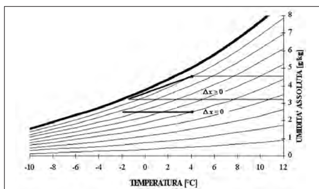
Figura 14. Trasformazioni dell'aria sulla batteria evaporante per diversi valori di umidità relativa.
