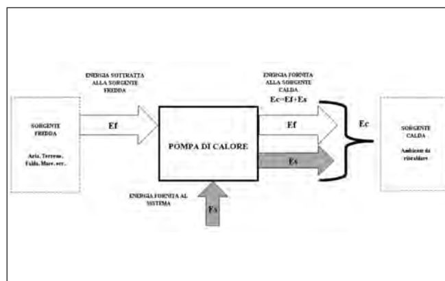
Figura 6. Bilancio energetico di un sistema a pompa di calore.
