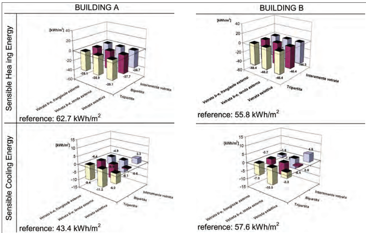
Figura 3. Risultati dei calcoli, differenze tra l'energia sensibile per il riscaldamento e il raffrescamento. Figura 4. Risultati dei calcoli, fabbisogno specifico di energia per il riscaldamento e il raffrescamento, edificio A.
