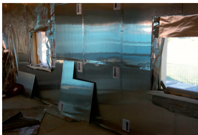
Figura 16. L'installazione dello strato di PCM.
