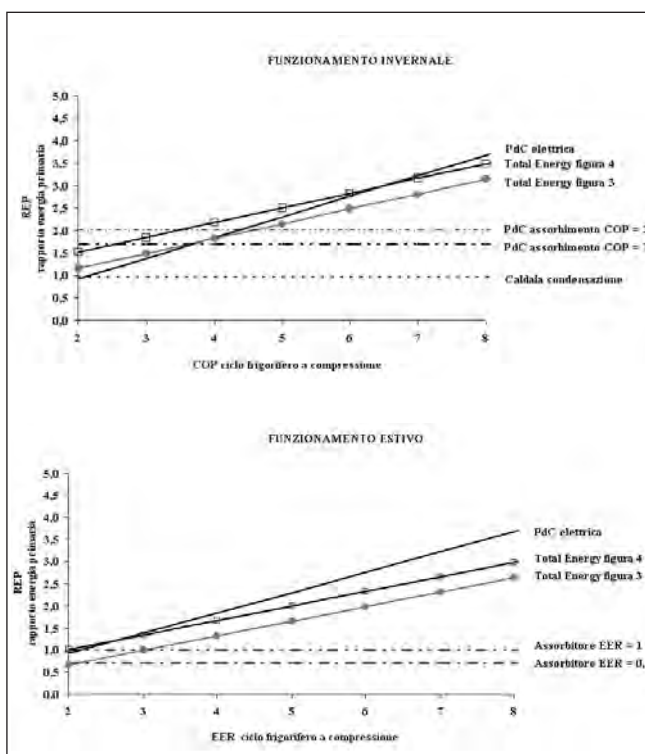
Figura 9. Valori di REP in funzionamento invernale ed estivo per i vari sistemi. Sistemi Total Energy : \eta_M = 0,33 , \eta_T = 0,5 , EER_{AS} = 0,7 , COP_{AS} = 1,7 .
