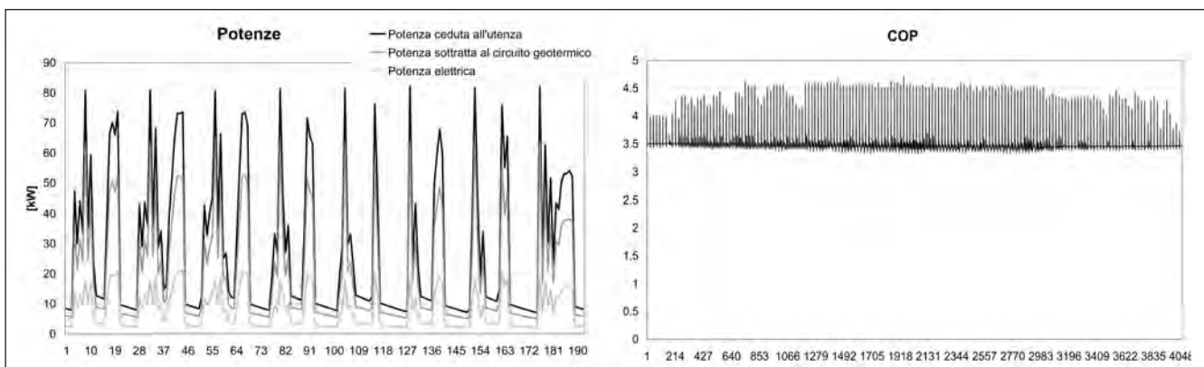
Figura 3. Profilo orario della potenza termica fornita (ceduta all'utenza), sottratta al terreno (circuiti geotermico) e della potenza elettrica assorbita di una pompa di calore geotermica a servizio di un piccolo edificio residenziale multifamiliare per alcuni giorni invernali; profilo orario del COP della medesima pompa di calore lungo tutta la stagione di riscaldamento.
