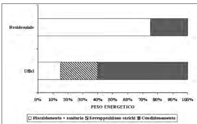
Figura 23. Ripartizione percentuale del consumo di energia in un anno (città del Nord Italia).
