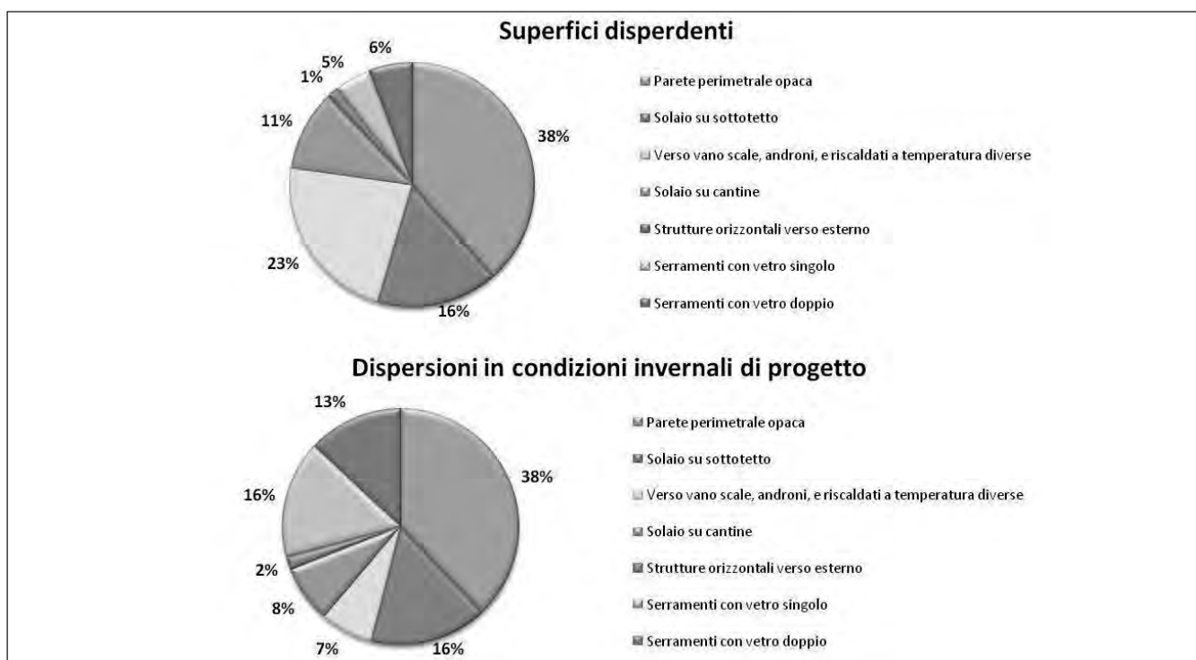
Figura 7. Confronto fra incidenza superficiale e della potenza termica dispersa in condizioni di progetto dei vari componenti di involucro edilizio.
