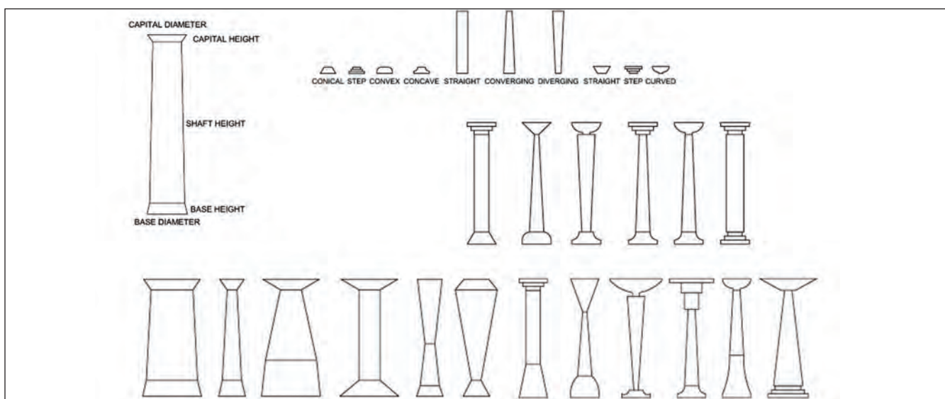
Figura 6. Studio parametrico degli elementi e le possibilità per il tipo "colonna".
