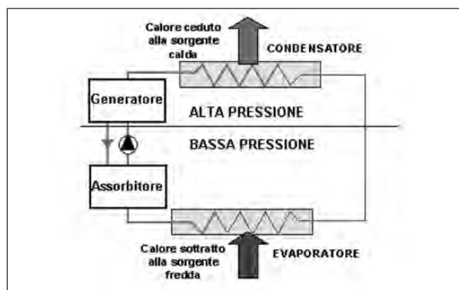
Figura 5. Ciclo frigorifero ad assorbimento.
