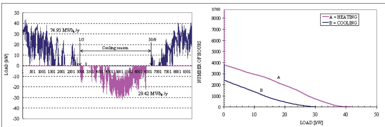
Figura 2. Profilo orario lungo un intero anno (8760 ore) dei carichi termici e frigoriferi di un edificio residenziale multipiano e curve di frequenza cumulata dei carichi (da E. Fabrizio, V. Corrado, M. Filippi, A model to design and optimize multi-energy systems in buildings at the design concept stage , in «Renewable Energy», vol. 35, n° 3 (2010) pp. 644-655).
