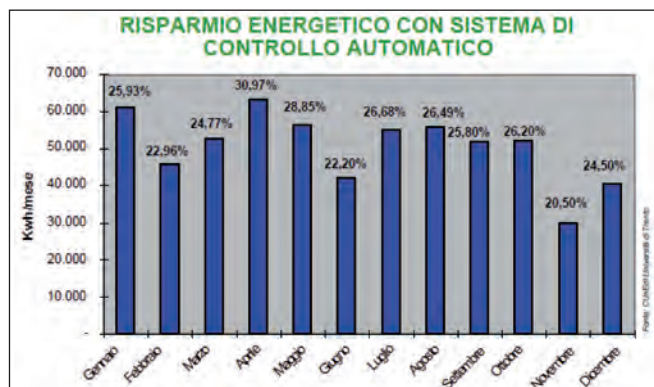
Figura 9. Risparmi energetici conseguiti in un edificio museale attraverso l'installazione di un sistema di building automation (da www.konnex.it).
