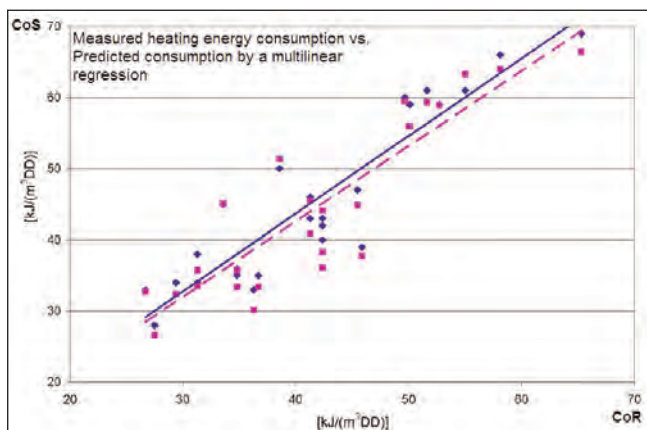
Figura 9. Esempio di correlazione tra indice di consumo specifico normalizzato rispetto ai gradi giorno invernali (DD = Degree Days) ottenuto da dati misurati (indice CoR, asse X) e stimati attraverso un modello predittivo (indice CoS, asse Y).
