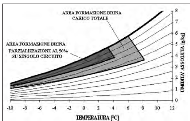
Figura 15. Area di formazione di brina sulle batterie evaporanti.
