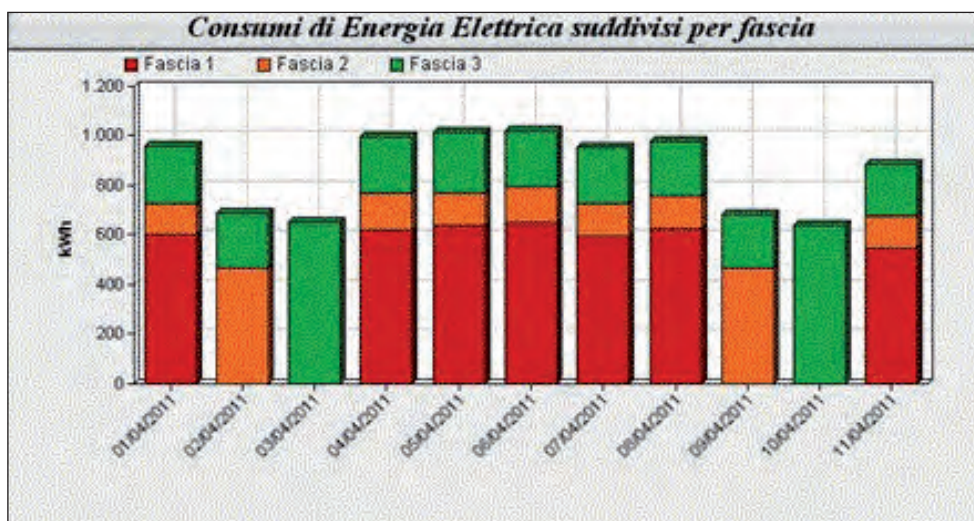
Figura 5. Andamento consumi elettrici di un dipartimento per fasce nei primi giorni del mese.
