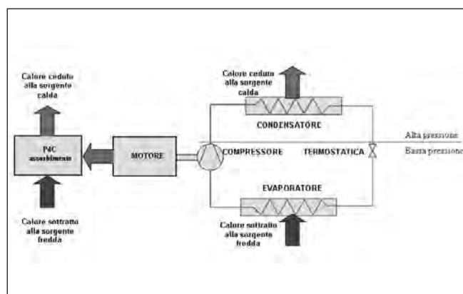
Figura 4. Sistema Total Energy nella configurazione più complessa (sistema di trigenerazione).
