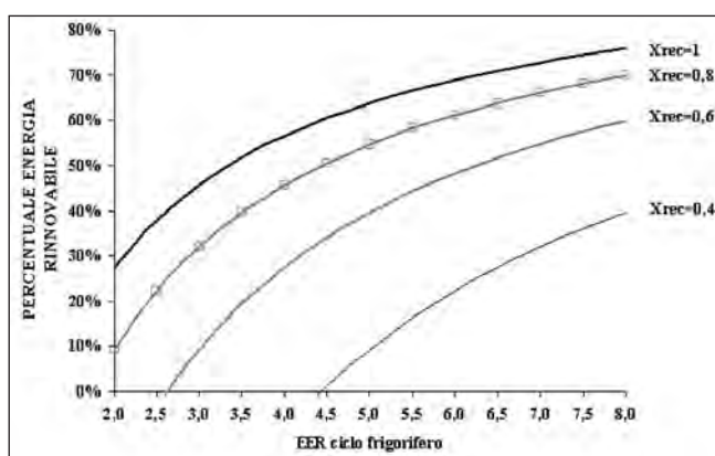
Figura 11. Percentuale di energia rinnovabile in funzionamento estivo: pompe di calore con compressore elettrico.
