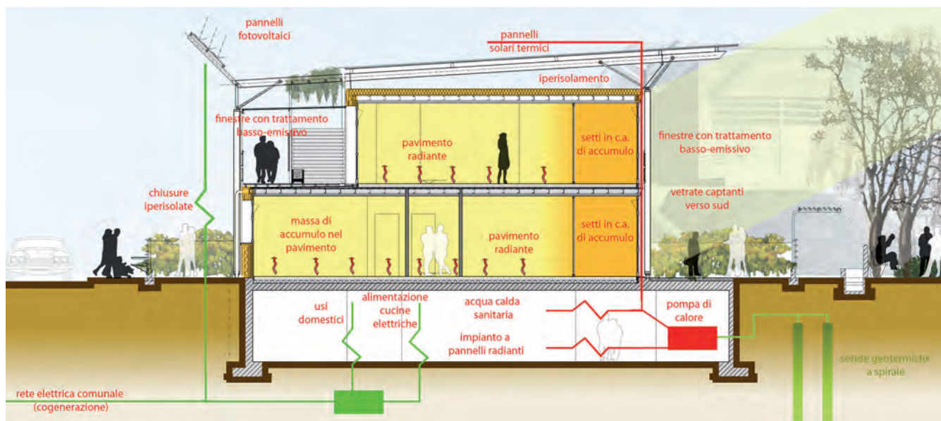
Figura 8. Funzionamento estivo; progetto B.I.R.D., Brescia: strategie per il risparmio energetico in estate (fonte: AIACE Srl).
