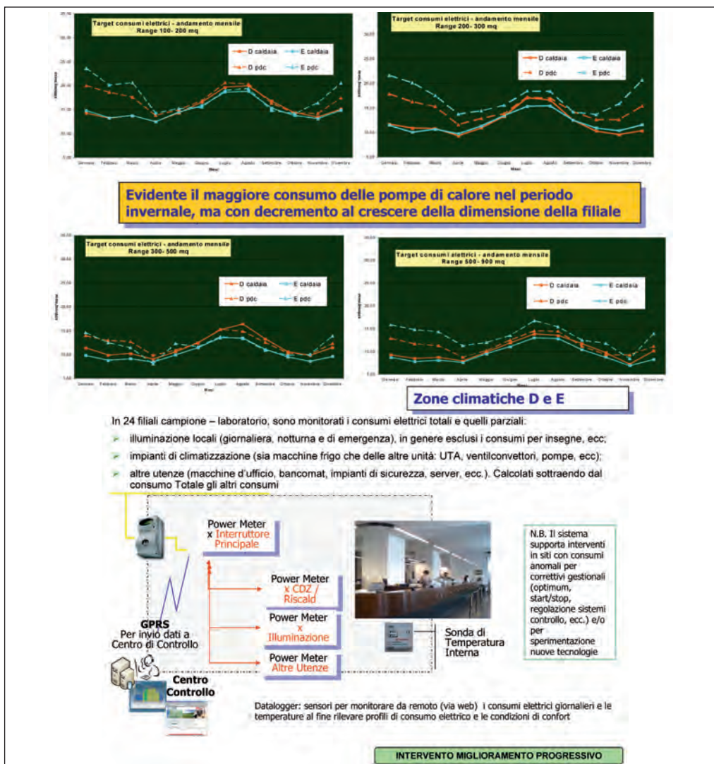
Figura 9b. Livello 3. ISP e Banche Rete: monitoraggio dei consumi elettrici e della temperatura via web - laboratorio (CSR – Energy Manager).
