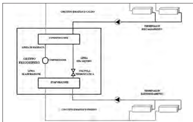
Figura 16. Recupero di calore da ambienti interni con gruppo frigorifero polivalente.
