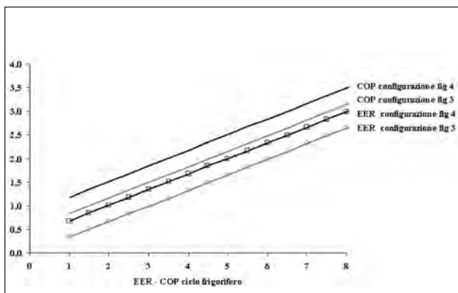
Figura 7. EER e COP dei sistemi Total Energy : \eta_M = 0,33 , \eta_T = 0,5 , EER_{AS} = 0,7 , COP_{AS} = 1,7 .
