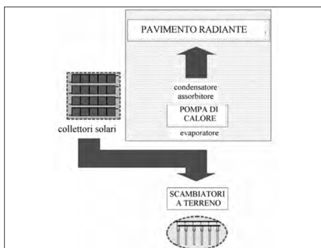
Figura 22. Fase estiva: i collettori solari ricaricano il terreno.
