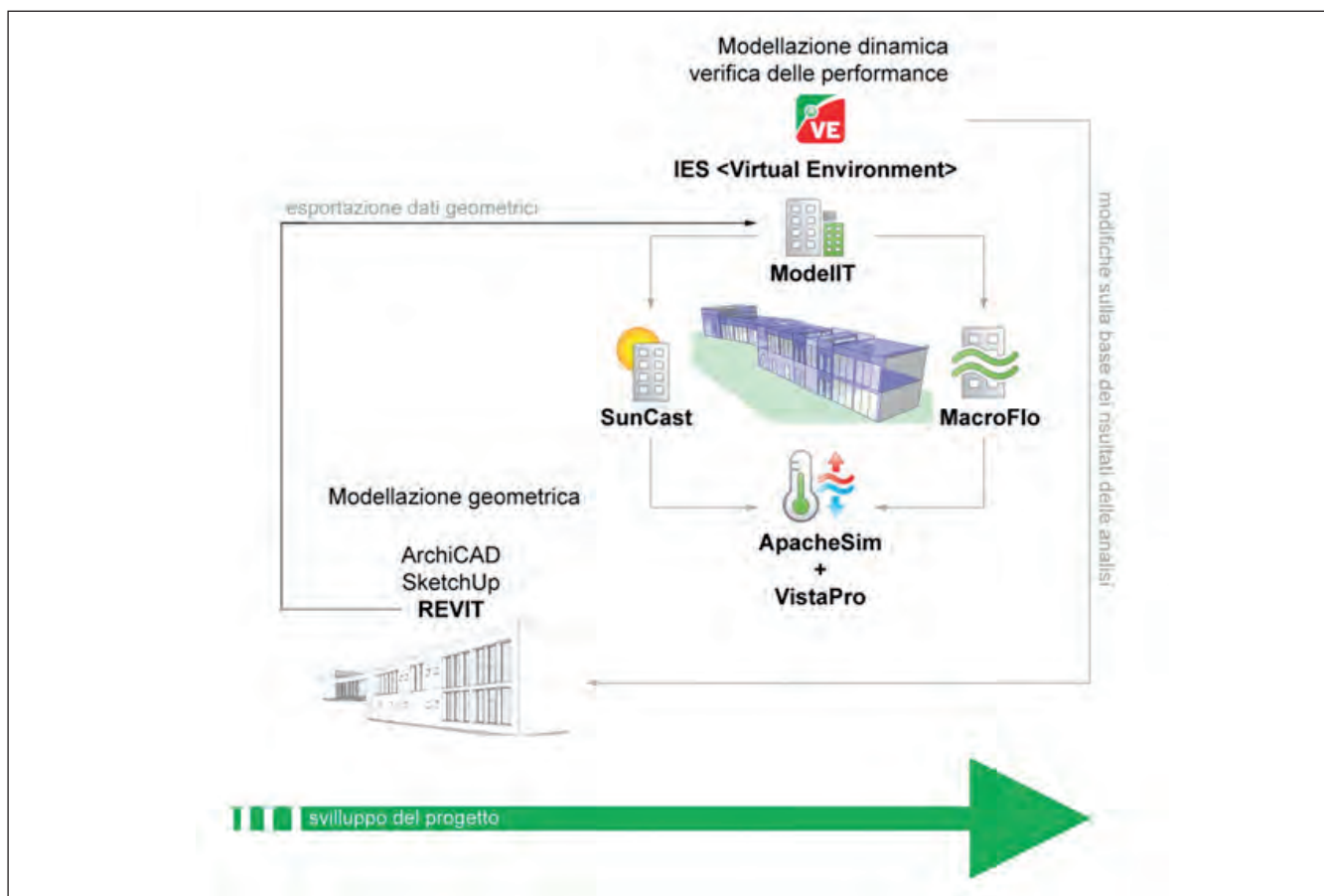
Figura 12. Flusso di lavoro ed informazioni con il software IES VE, all'avanzare del processo progettuale.
