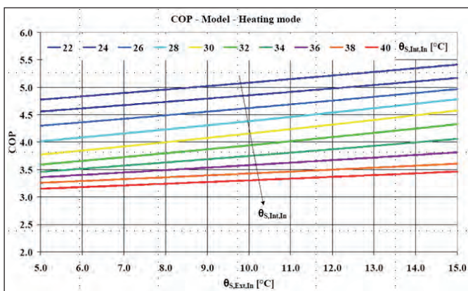
Figure 1a, 1b. Esempi di andamenti del coefficiente di effetto utile per pompe di calore acqua-acqua in modalità di riscaldamento (a) e raffrescamento (b), al variare delle temperature del fluido esterno ( \theta_{S,Ext,In} ) e del fluido interno ( \theta_{S,Int,In} ).
