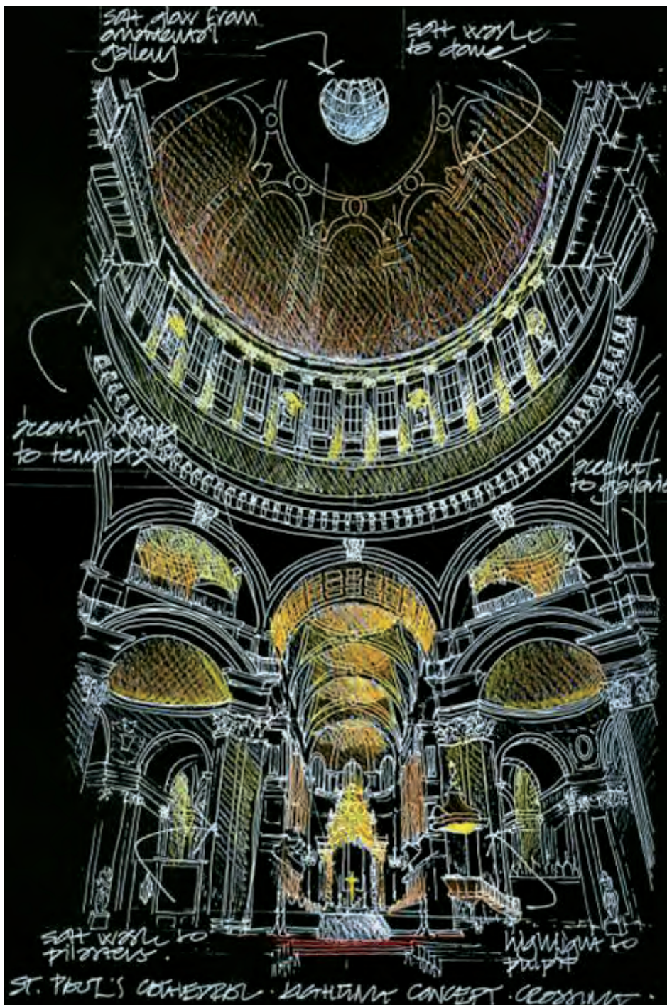
Figura 1. Rappresentazione mediante disegno a mano libera dell'idea di progetto della luce (Speirs and Major Associates, St. Paul's Cathedral, Londra [9]).
