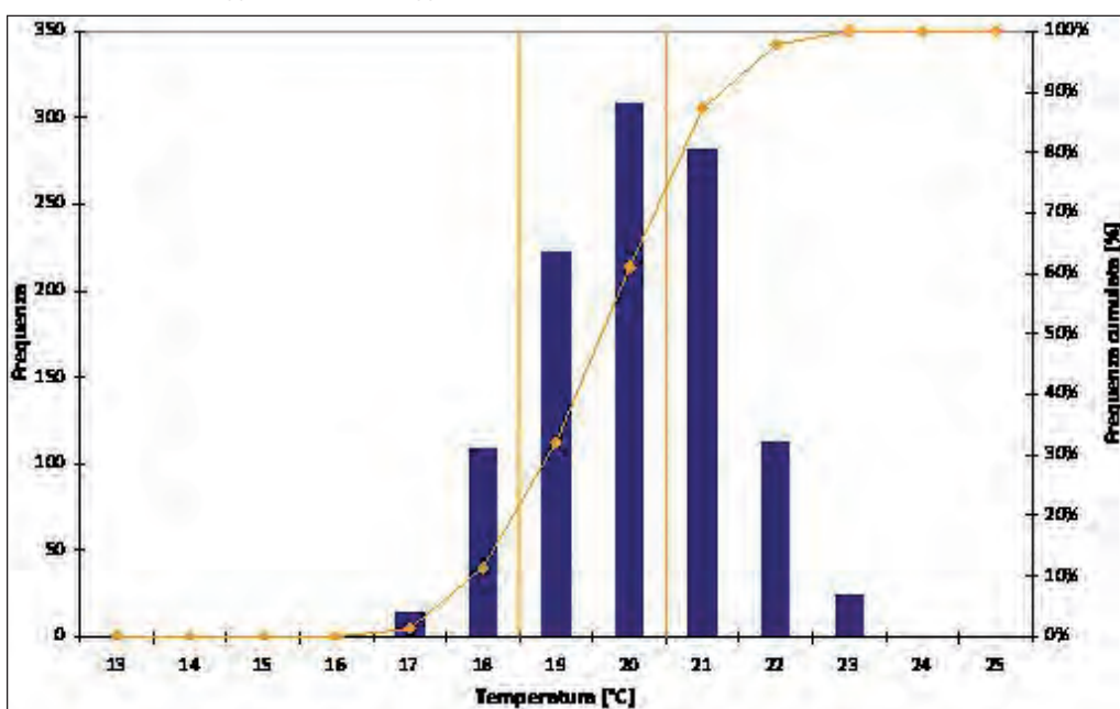
Figura 11. Distribuzione in frequenza e frequenza cumulata dei dati di temperatura interna rilevati all'interno di uno dei locali oggetto di monitoraggio ambientale.
