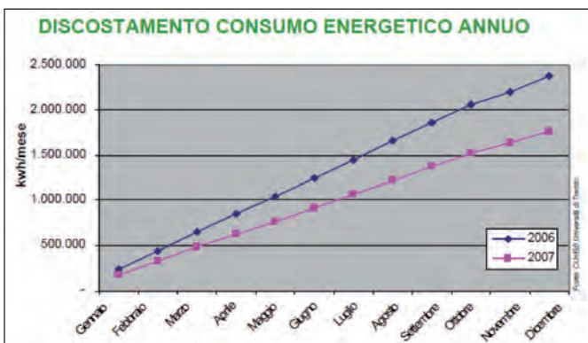
Figura 8. Scostamento del consumo energetico annuo di un edificio museale prima (2006) e dopo (2007) l'installazione di un sistema di building automation (da www.konnex.it).
