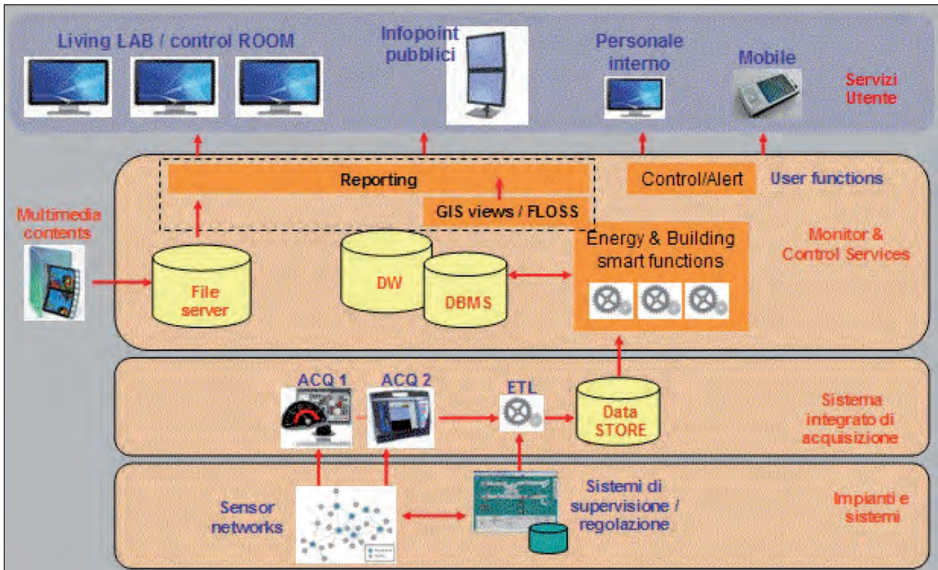
Figura 3. Il Living LAB del Politecnico di Torino.
