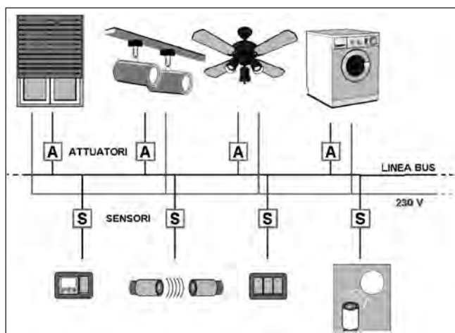
Figura 1. Esempio di architettura di un sistema BUS.
