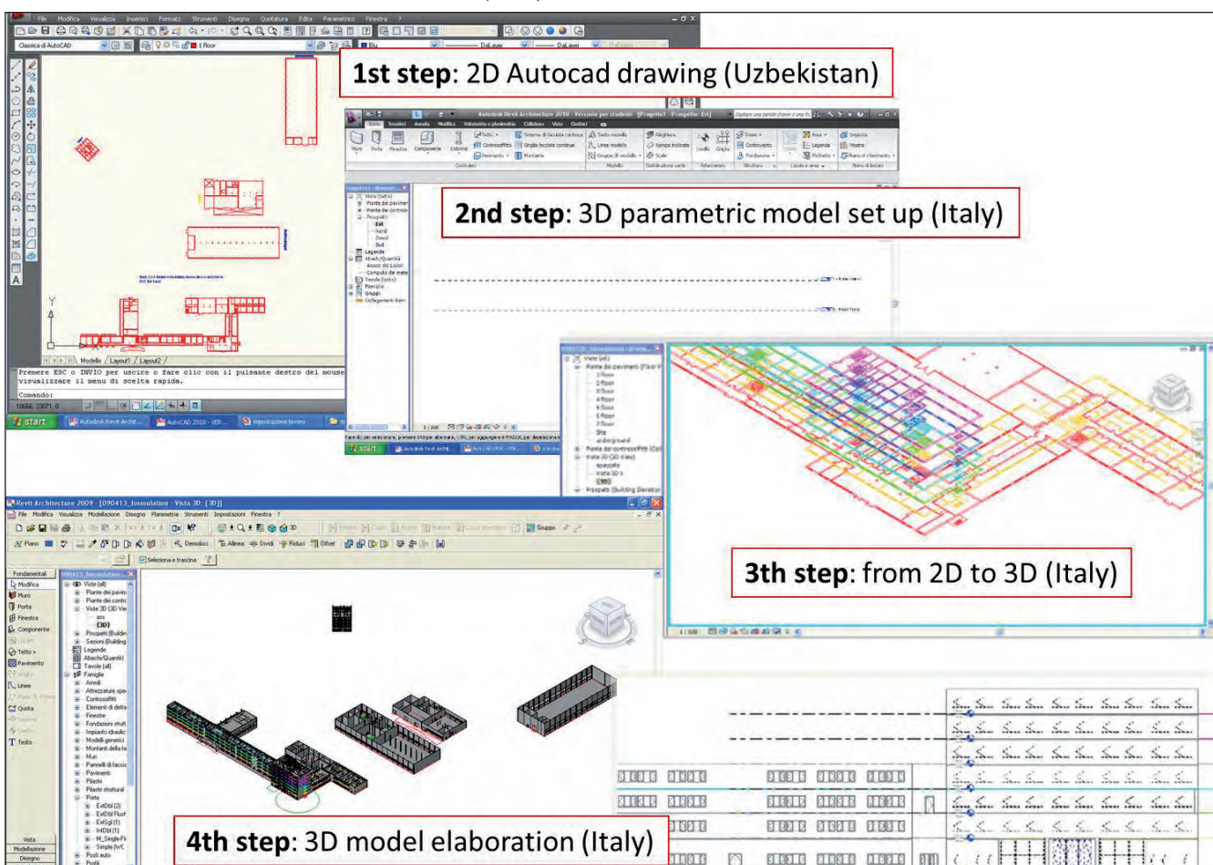
Figura 2. Masterplan modellato con oggetti generici di tipo parametrico a partire da file CAD bidimensionali della sede della Turin Politecnica Universitari di Tashkent in Uzbekistan. Autore: A.Osello (2009).
