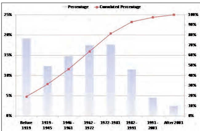
Figura 6. Distribuzione degli edifici di un campione in funzione del valore del medio della trasmittanza termica U [W/m 2 K] (asse X) dei componenti di involucro trasparente: frequenza percentuale su asse Y.
