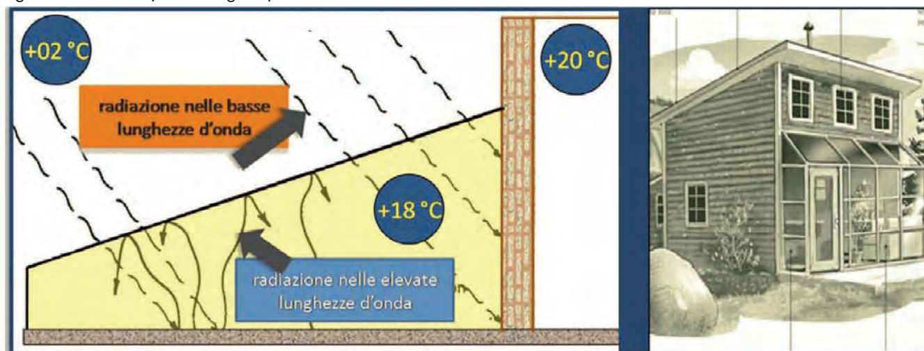
Figura 6. Serre Solari: fenomenologia di funzionamento
