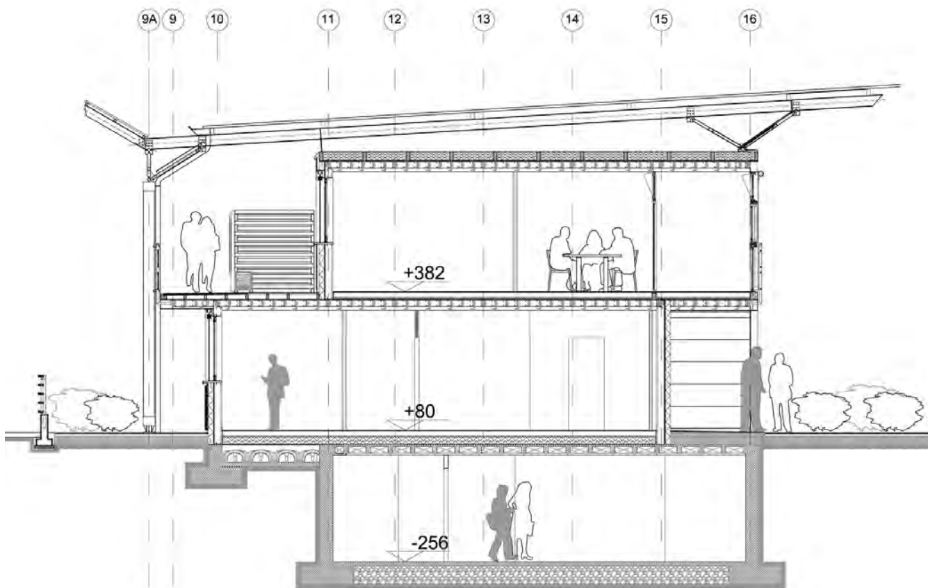
Figura 9. Sezione trasversale dell'edificio B; progetto B.I.R.D., Brescia: sezione di dettaglio dell'edificio residenziale, costruito con tecnologie a secco S/R (fonte: AIACE Srl).
