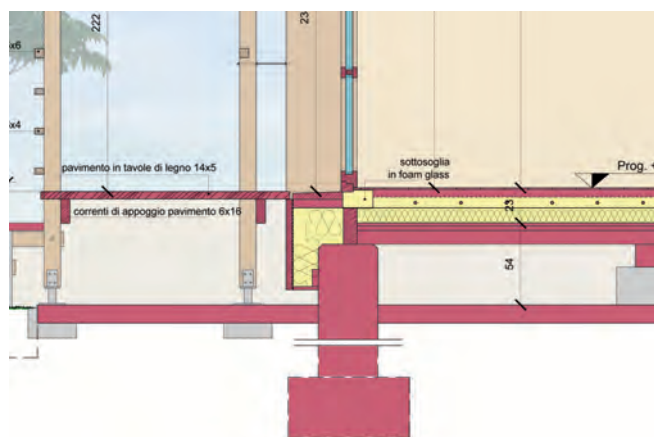
Figura 14. L'attacco a terra: uso di foam glass sottosoglia.
