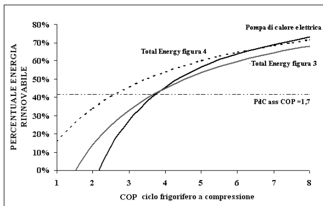
Figura 10. Percentuale di energia rinnovabile in funzionamento invernale per i vari sistemi. Sistemi Total Energy: \eta_M = 0,33 , \eta_T = 0,5 , COPAS = 1,7.
