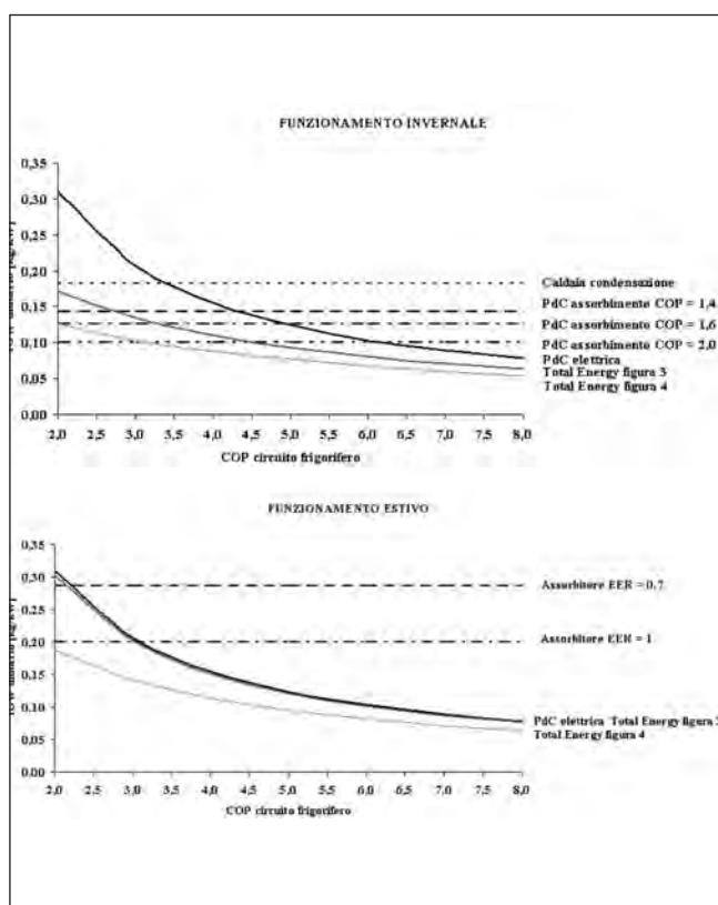
Figura 12. Emissioni di CO 2 per kWh termico prodotto.
