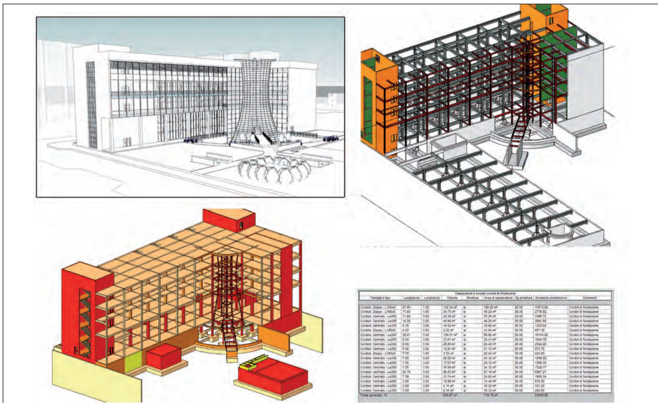
Figura 8. Vista concettuale dell'Energy Center, modelli strutturali e abaco per il calcolo delle cassetture. Autori: G. Cangialosi e M. Lo Turco (2011).
