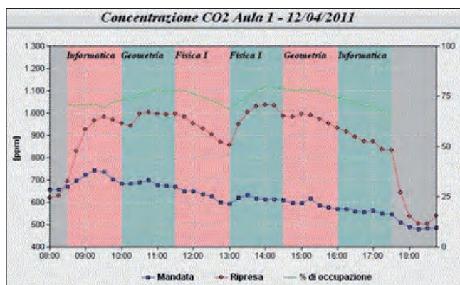
Figura 8. Monitoraggio occupazione aule tramite variazione percentuale CO 2 .
