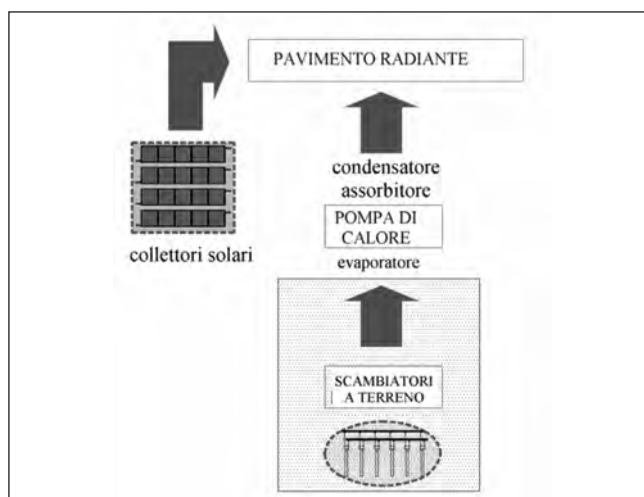
Figura 20. Riscaldamento diretto da collettori solari con il contributo della pompa di calore con sorgente fredda terreno.
