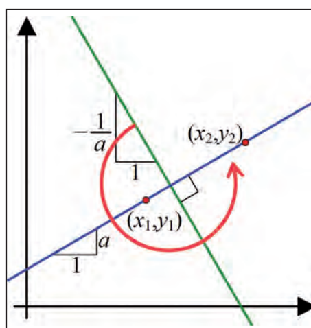
Figura 1. I parametri della finzione di una retta concorrono a descrivere tutto lo spazio piano.
