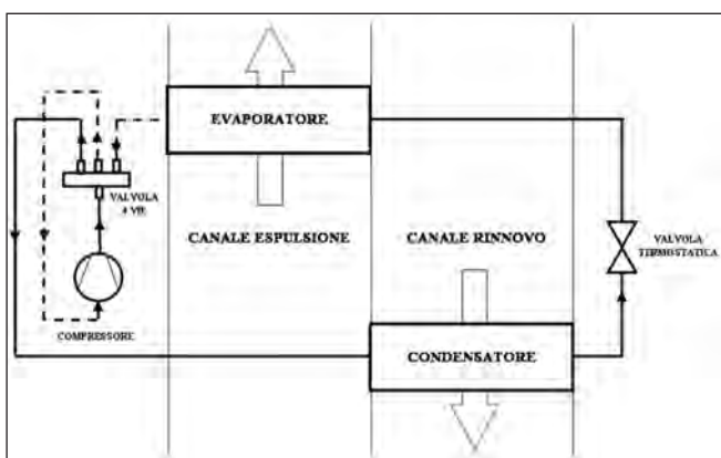
Figura 18 b. Recupero tramite pompa di calore a compressione (funzionamento invernale).
