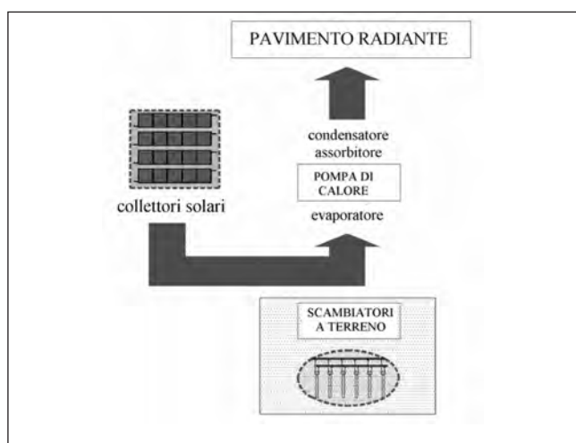
Figura 21. I collettori solari alimentano l'evaporatore della pompa di calore.
