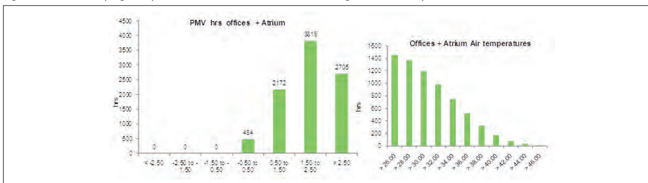
Figura 5. Valutazione progetto: qualità dell'ambiente interno, PMV e Ta negli ambienti occupati.
