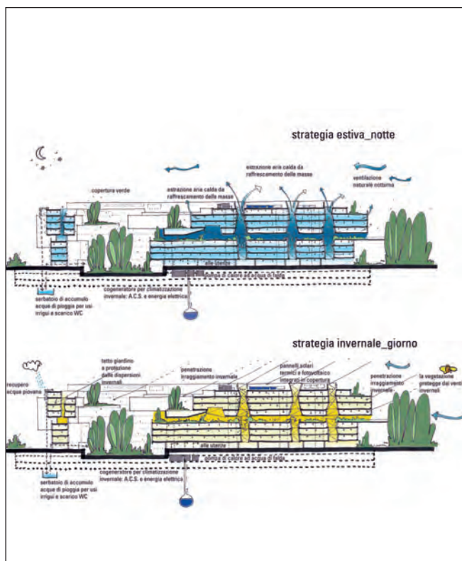
Figura 2. Mario Cucinella Architects, Campidoglio 2, Roma, Italia 2007 (esito di concorso).
