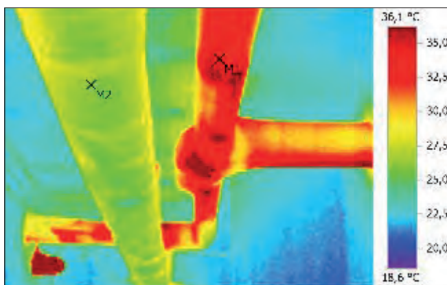
Figura 6. Termografia sulla rete di distribuzione del fluido termovettore.
