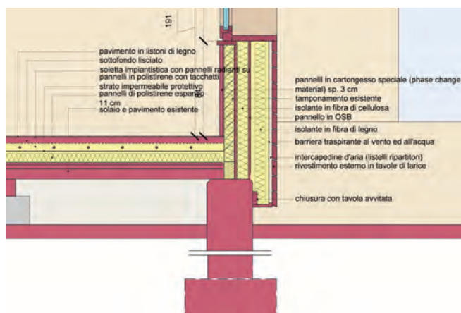
Figura 13. L'attacco a terra: il basamento della parete.
