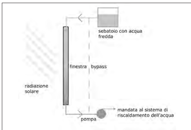
Figura 9. Principio di funzionamento del collegamento dell'intercapedine di una finestra con un circuito ad acqua.
