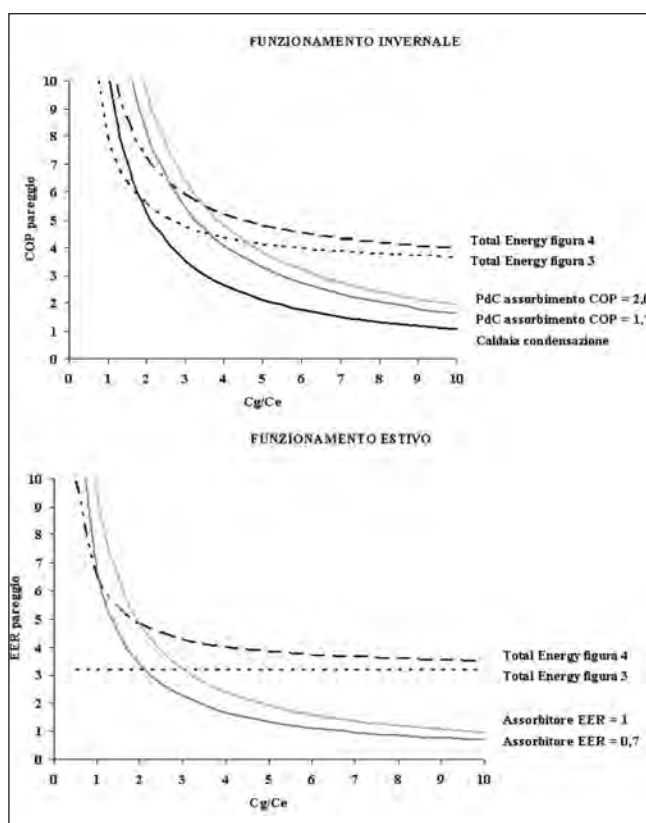
Figura 13. COP pareggio per una pompa di calore elettrica in funzione del rapporto tra costo del metano e costo dell'energia elettrica.
